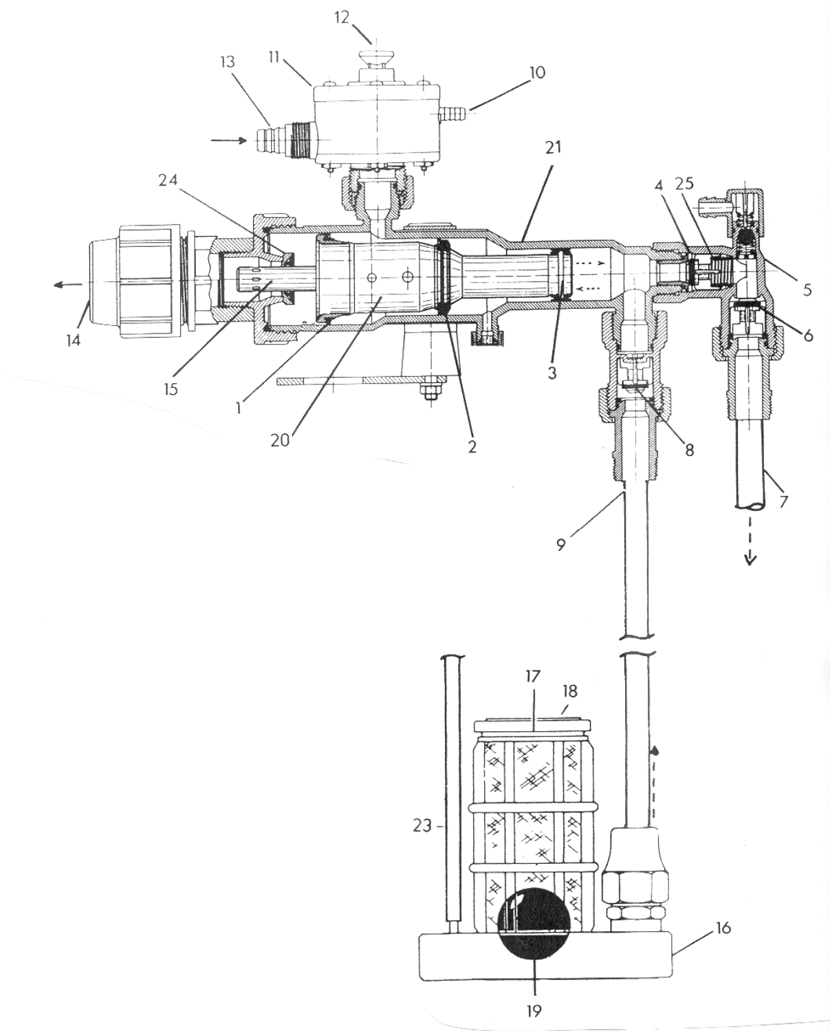
Obrázek č. 1 – PŘÍSLUŠENSTVÍ ČERPADLA (sací typ)
